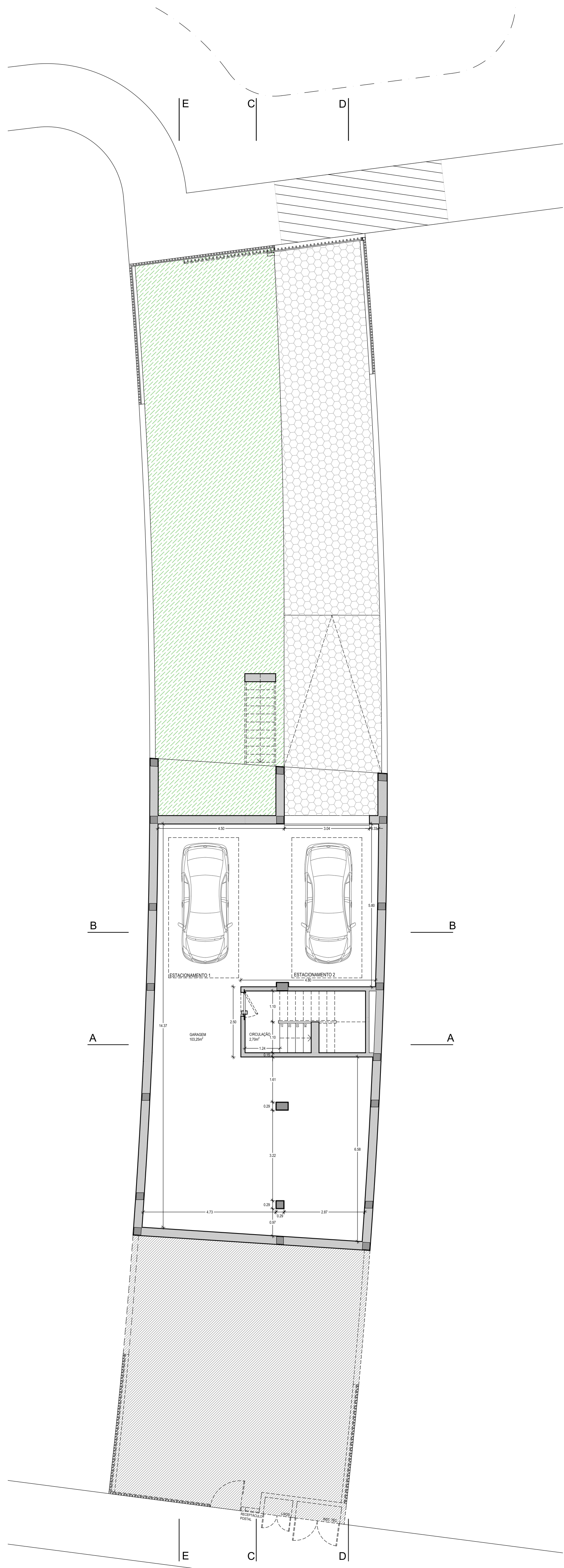
planta PISO -1
