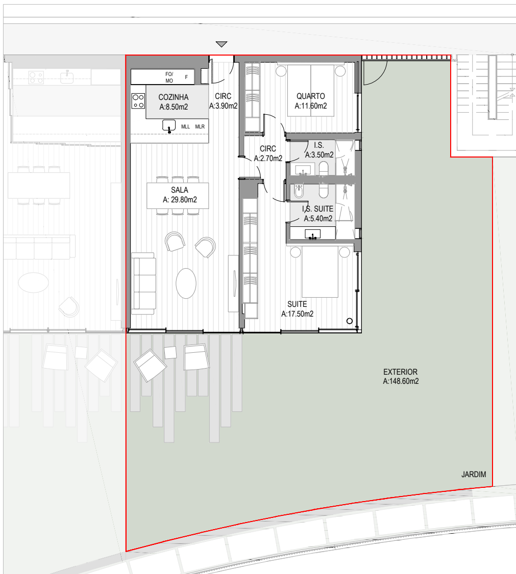
PLANTA | SEM ESCALA
