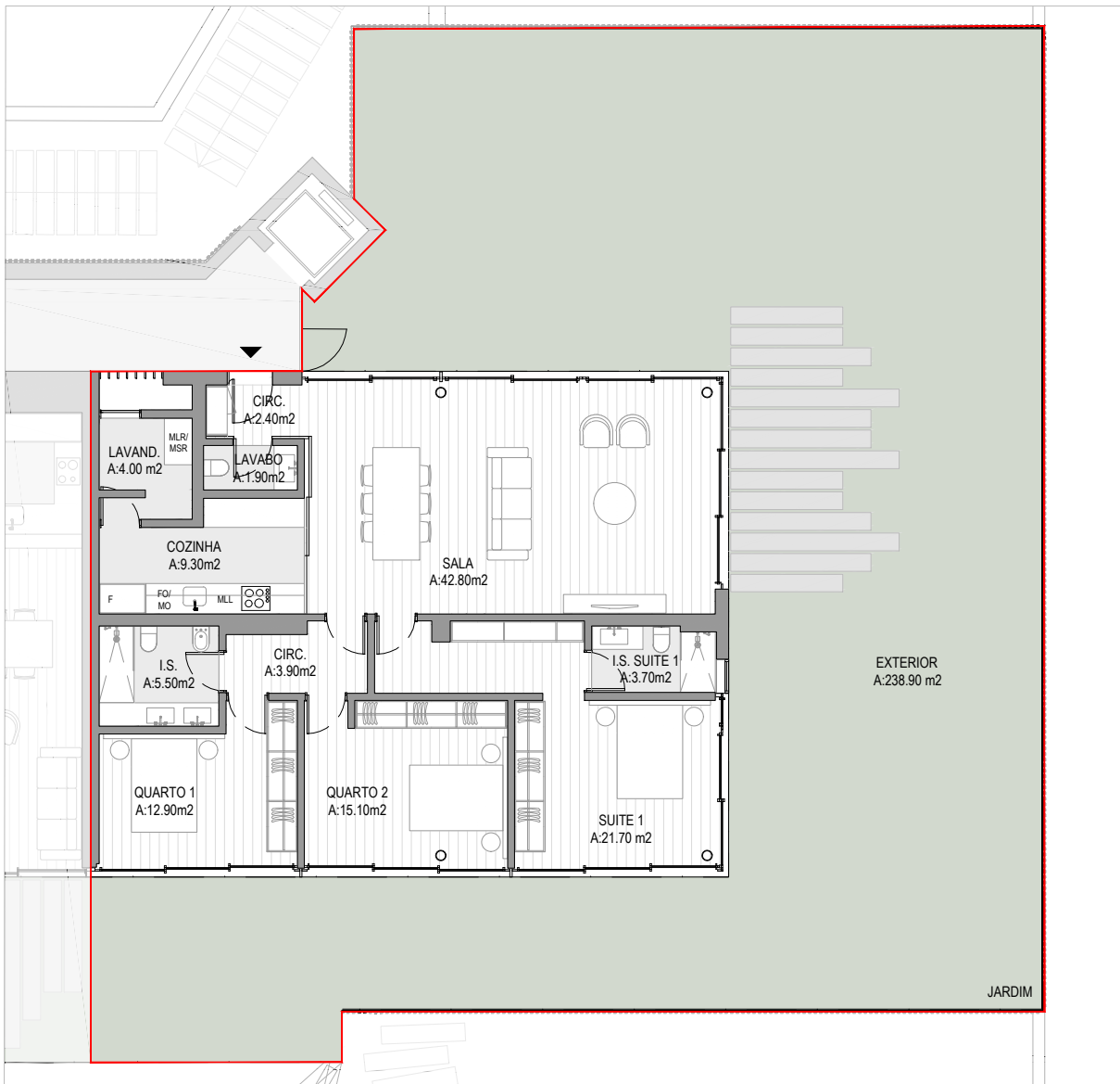
PLANTA | SEM ESCALA
