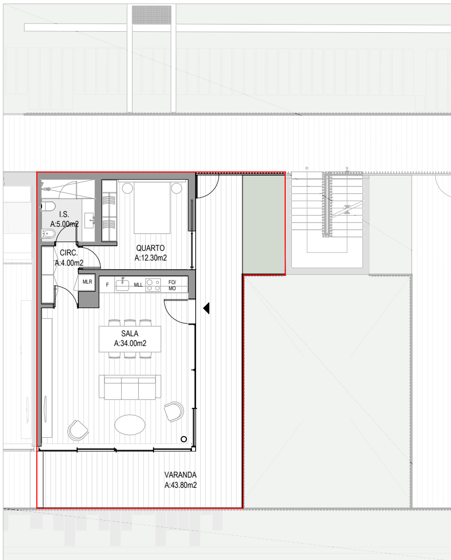
PLANTA | SEM ESCALA
