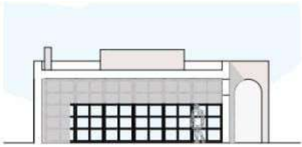
Corte DD
